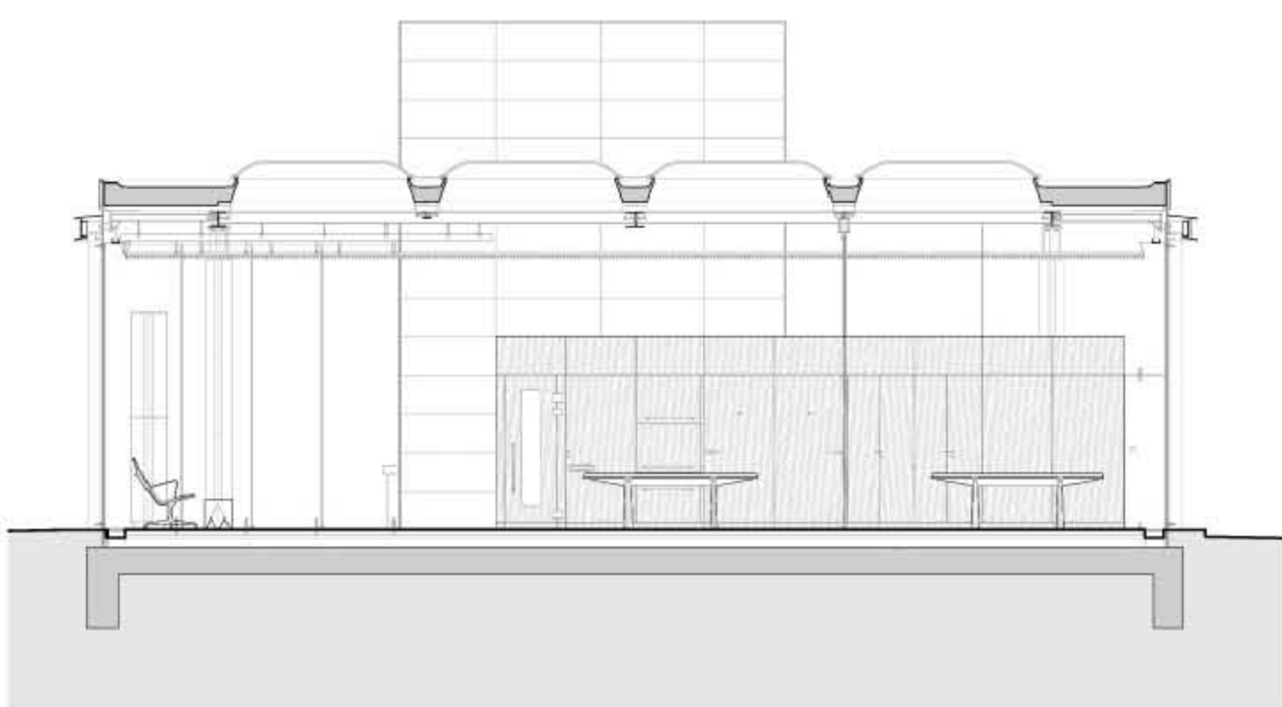
longitudinal Section
